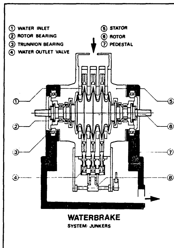
Fig. 3 Waterbrake
