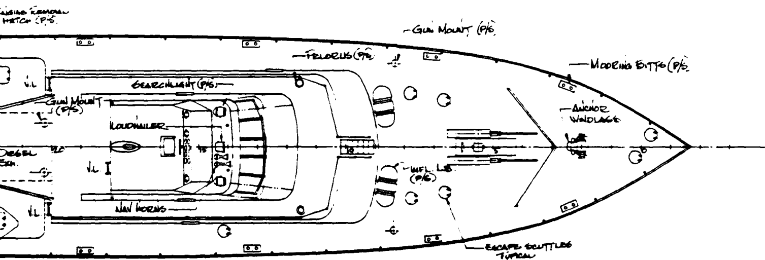
PLAN VIEW SCALE: \frac{1}{4} " = 1'-0"
