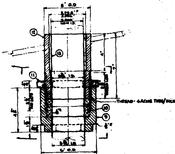
DET 66 STUFFING BOX SCALE: 6" = 1'-0"
