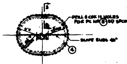
DET 3A NT. MANHOLE SCALE: 1 1/2" = 1'-0"
