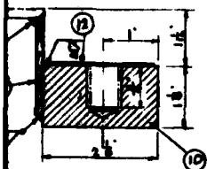
DET 5B SCALE: FULL SIZE
