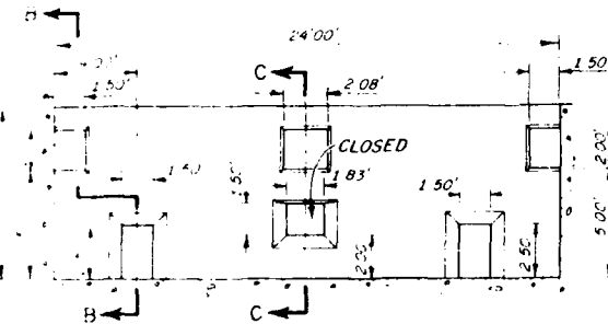
BAFFLE 249
