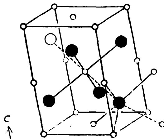
(b) CrS
