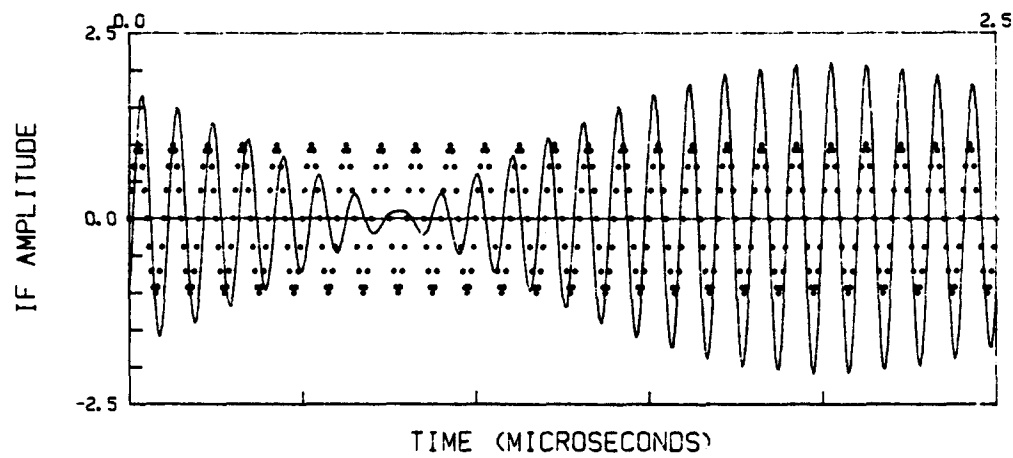
Figure A-10. IF Amplitude ( N=1.1S ).
