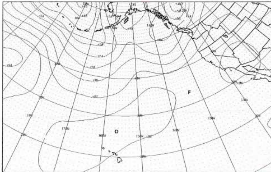
2B-35d. FNOc PE 500-mb Analysis. 1200 GMT 28 August 1981.
