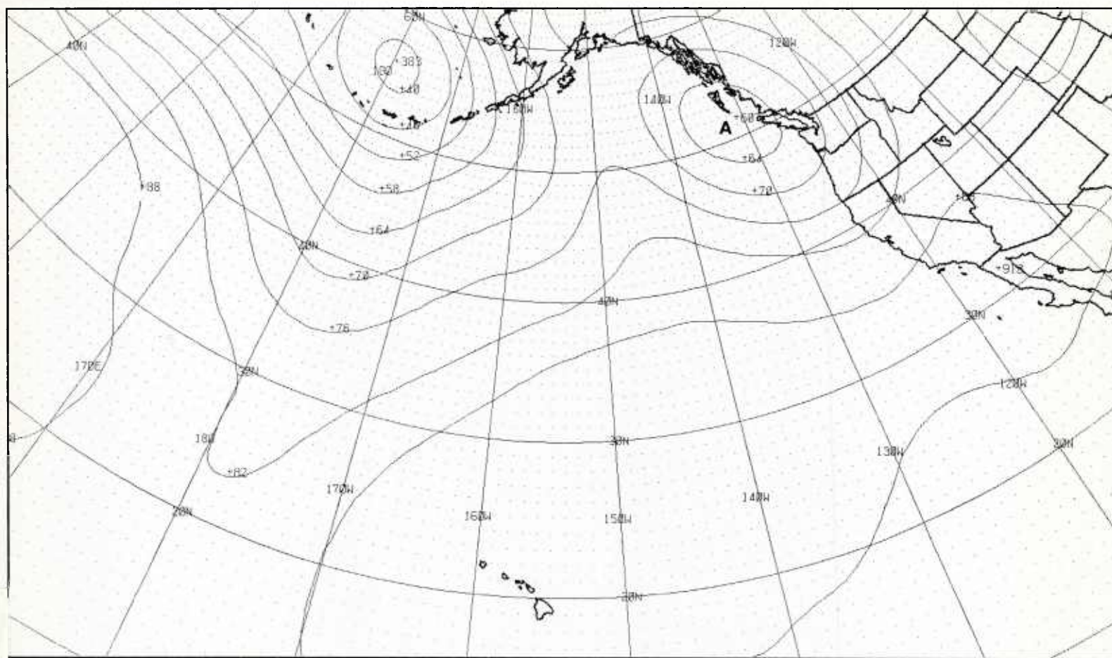
2B-29a. FNOC PE 24-hr 500-mb Prognosis. Valid 1200 GMT 27 August 1981.
