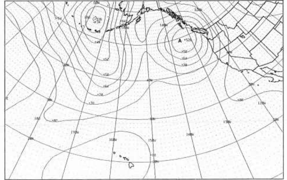
2B-27d. FNOC PE 500-mb Analysis. 0000 GMT 26 August 1981.
