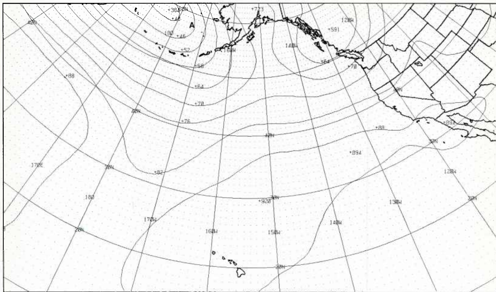
2B-33a. FNOC PE 24-hr 500-mb Prognosis. Valid 1200 GMT 28 August 1981.
