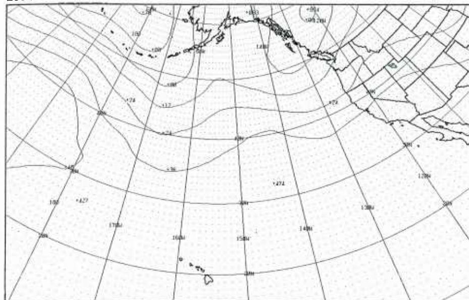
2B-35c. FNOc PE 200-mb Analysis. 1200 GMT 28 August 1981.
