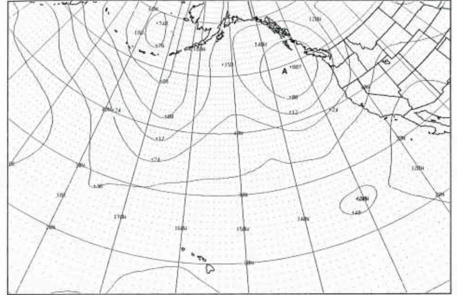
2B-27c. FNOC PE 200-mb Analysis. 0000 GMT 26 August 1981.
