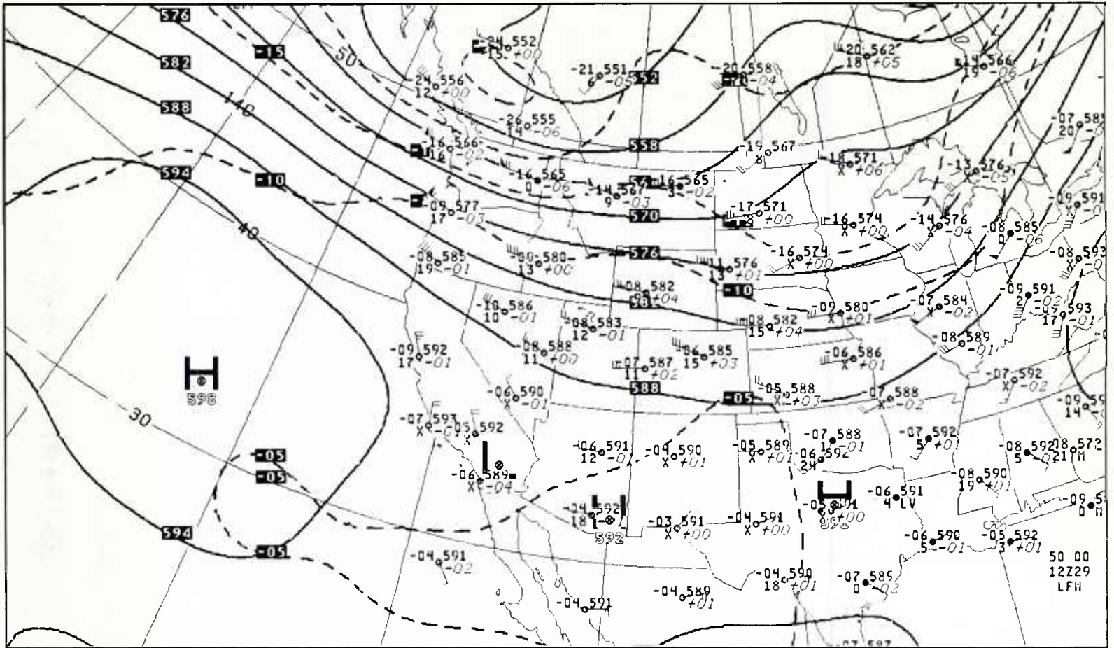
3B-11a. NMC 500-mb Analysis. 1200 GMT 29 August 1977.
