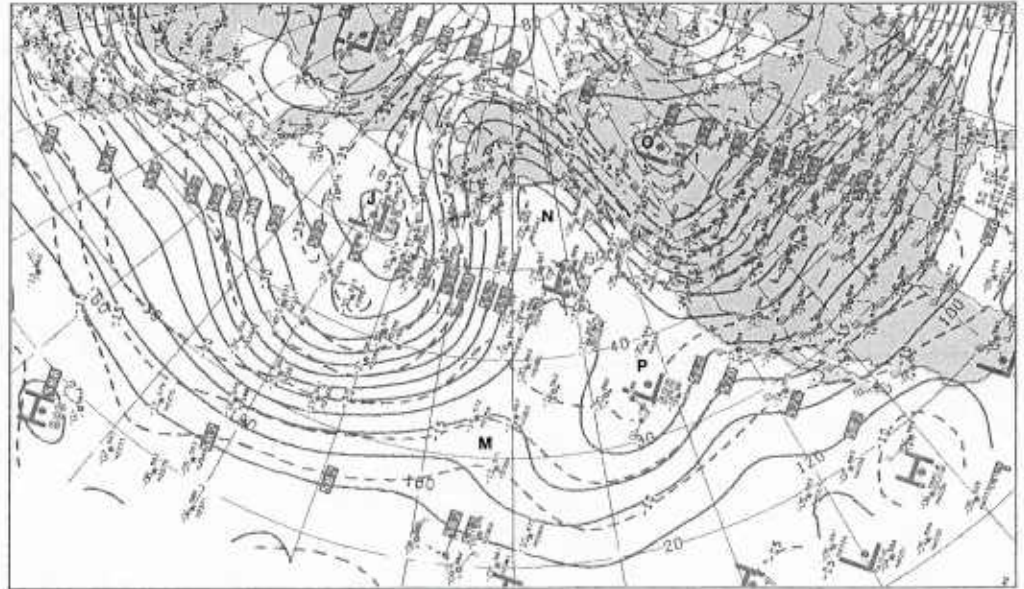
1B-18b. NMC 500-mb Analysis. 0000 GMT 28 December 1978.
