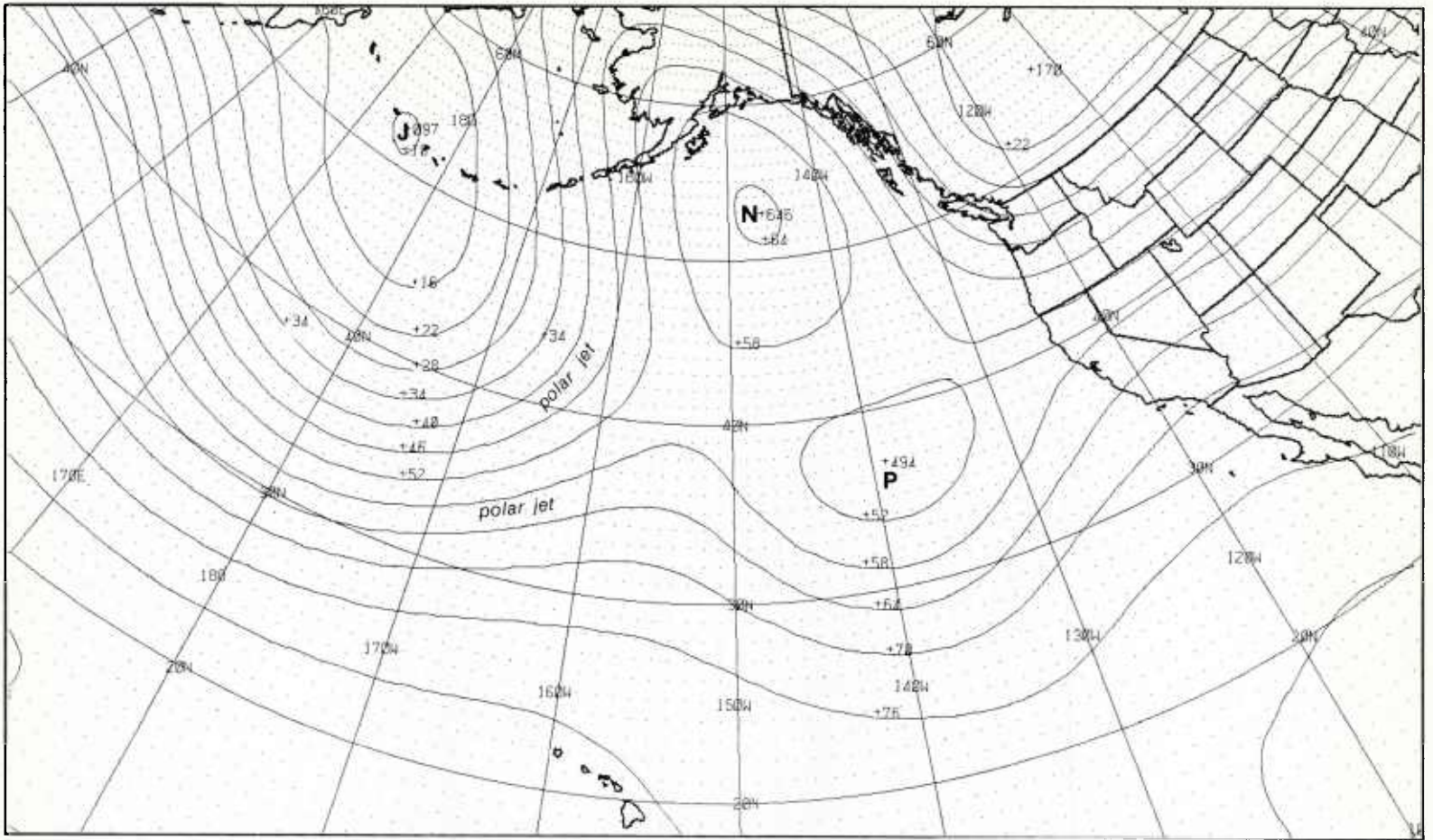
IB-17a. FNOC PE 36-hr 500-mb Prognosis. Valid 0000 GMT 28 December 1978.
