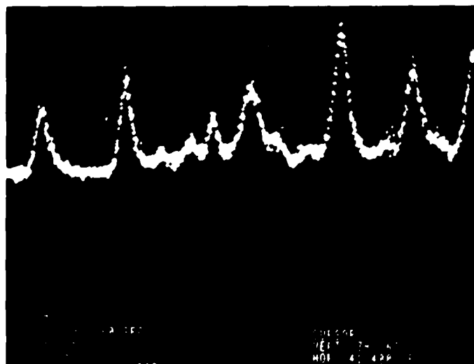
Figure G-4. Spectra 3200 - 3508 Å
