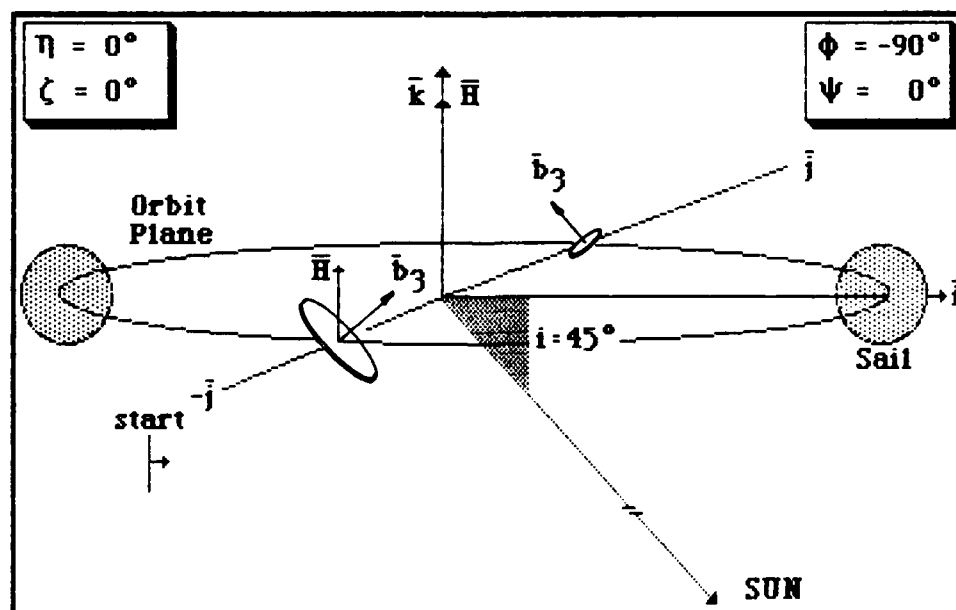
Fig. 4.4A: 45^\circ Inclination
