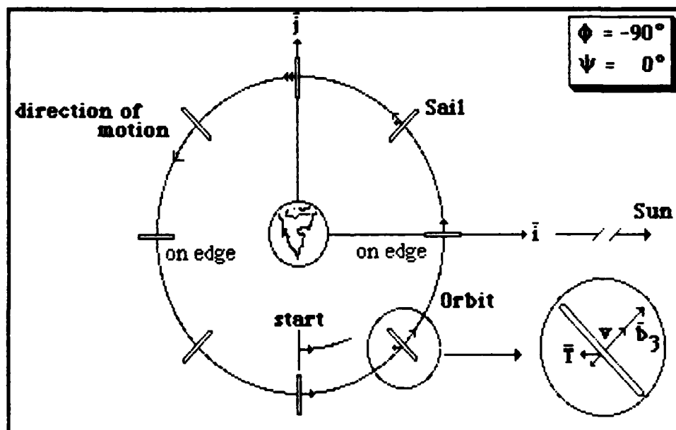
Fig. 4.3: 0^\circ Inclination
