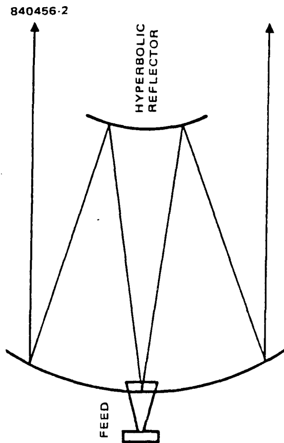
b) CASSEGRAIN
