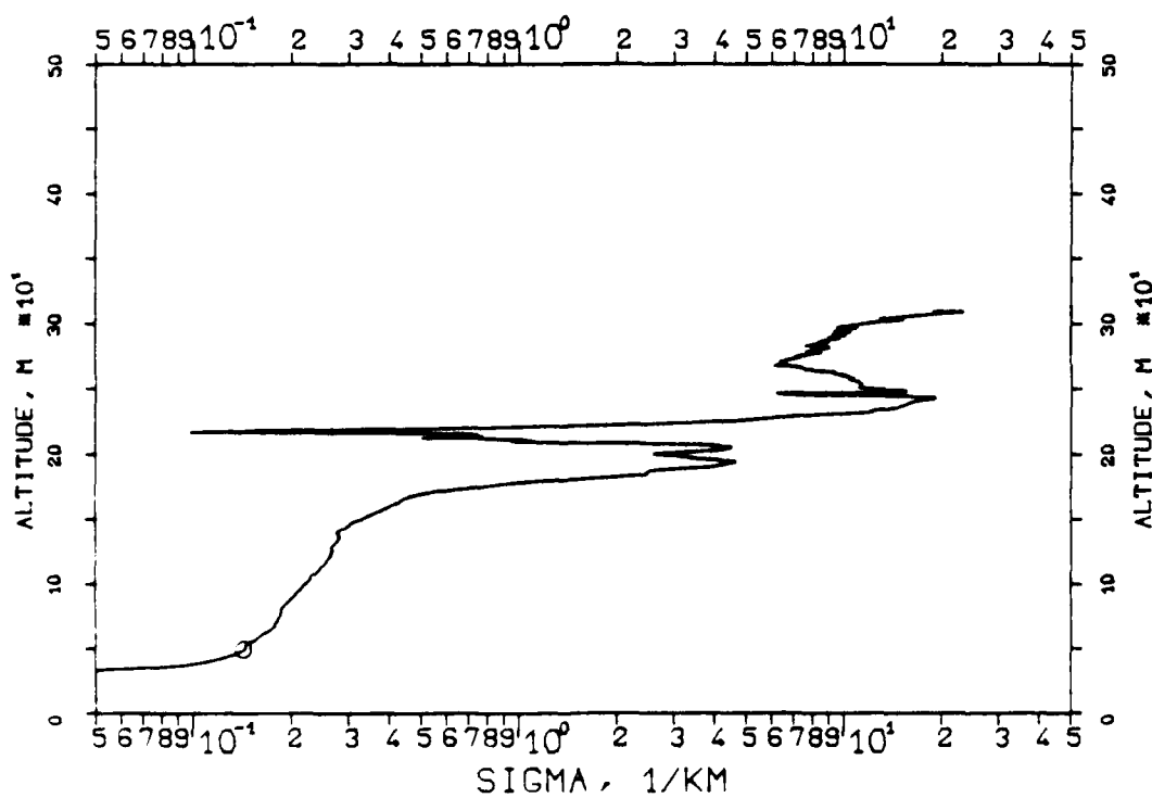
FIG. 7.24 KLETT-PROFILE, 0694NM, EL. 19DG12MN 821214, 16:47-16:48, CET RM=0.942KM, SM=20.0000/KM, K=1.000
