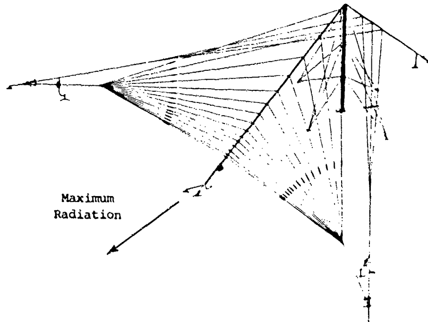
OE-85/86 antenna.
