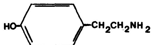
TYRAMINE
