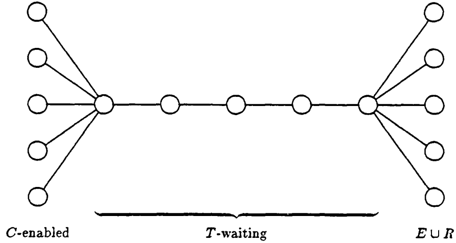
Figure 9: The relation <_q .
