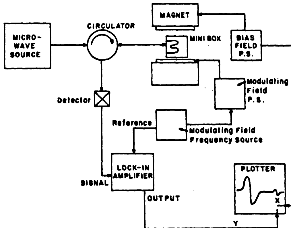
Fig. 2-1: FMR Apparatus
