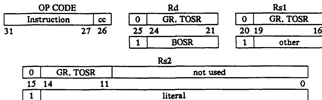
Fig. 5.1. Instruction format.
