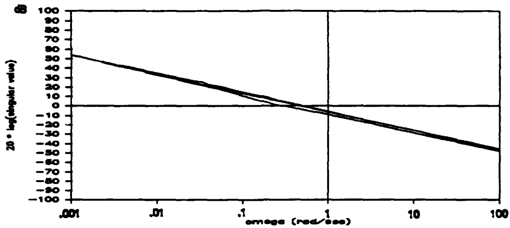
(d) Kalman Filter Loop, G_{KF}
