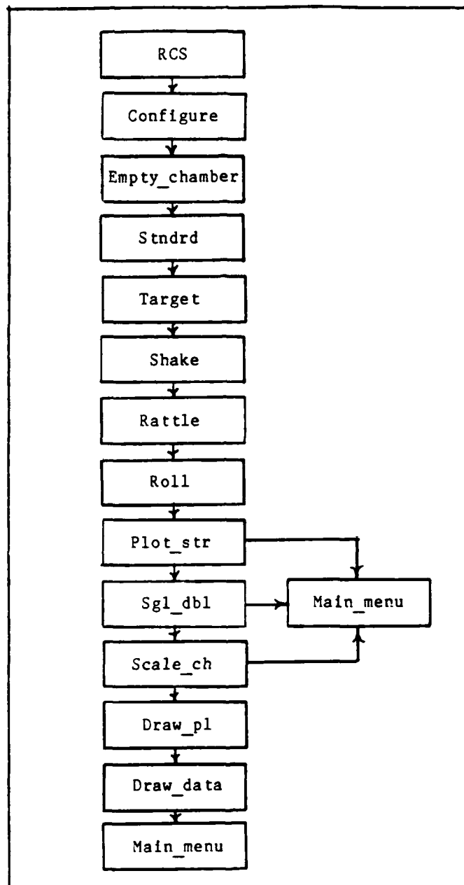
Fig. 20. Rcs Subroutine
