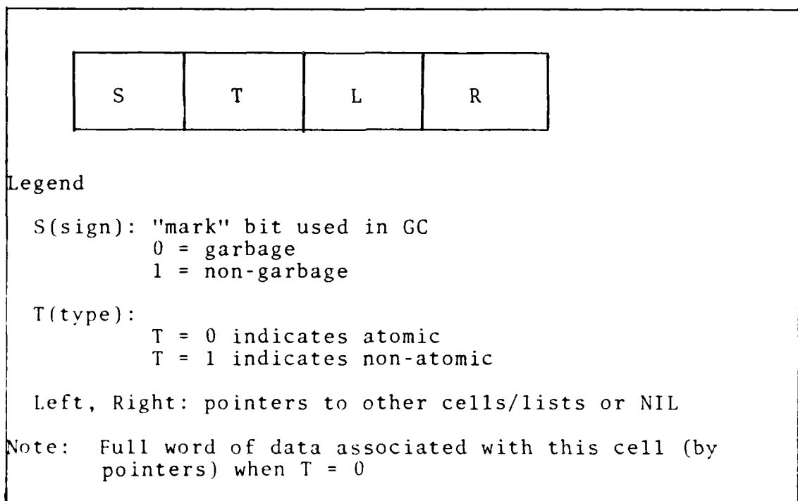
Figure 3.1 LISP Cell Format.
