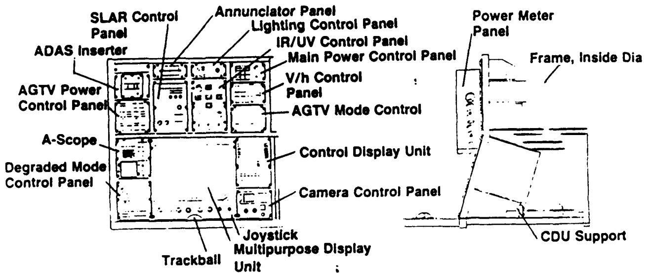
Figure 3-8. SSO Console
