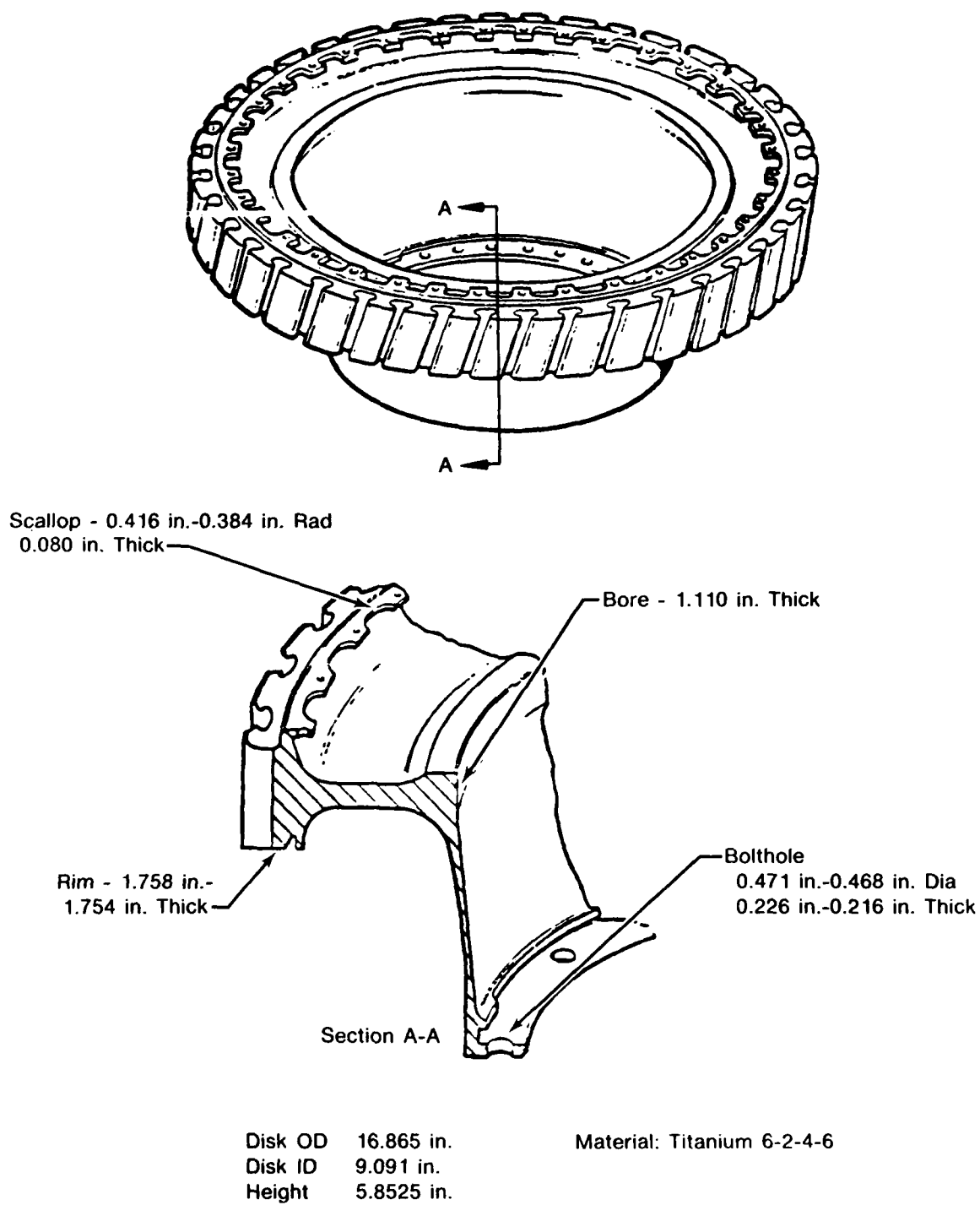
Figure H-3. 3rd-Stage Fan Disk (P/N 4048903)
