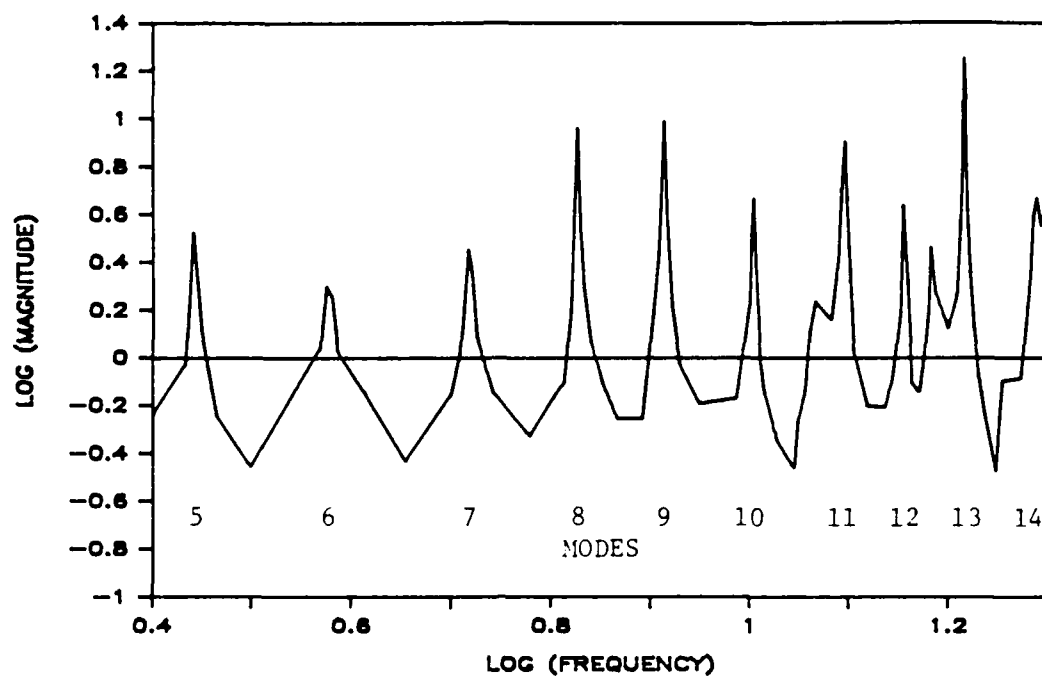
A: OPEN-LOOP
