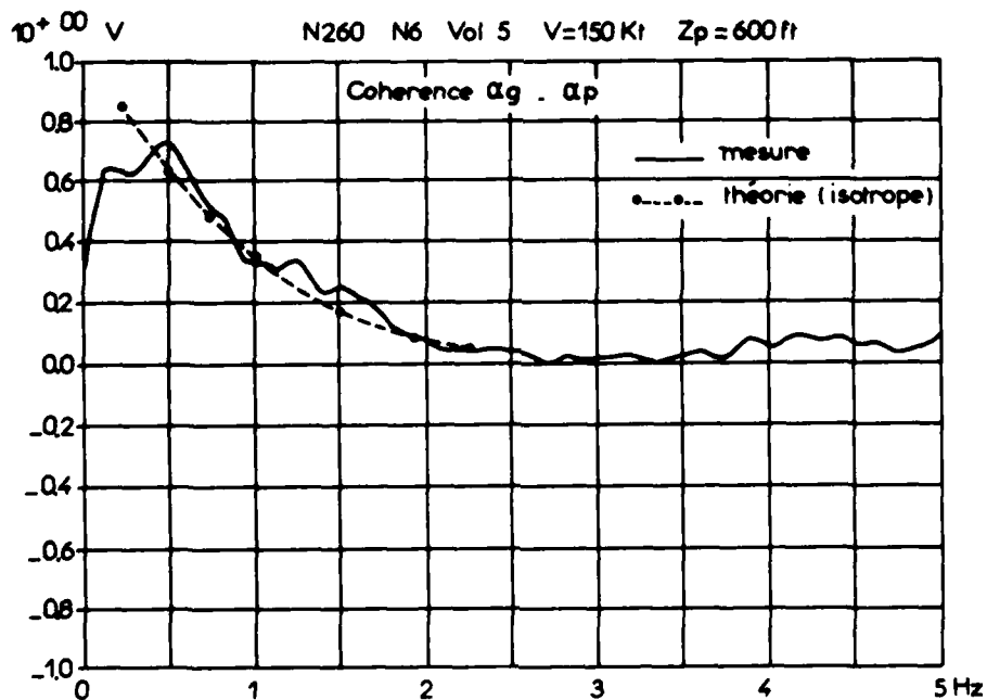
Fig.10 Cohérence entre la turbulence mesurée en 2 points
