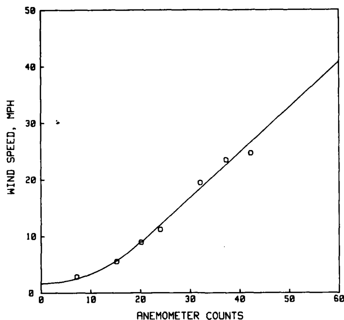
Fig. 3—Anemometer calibration
