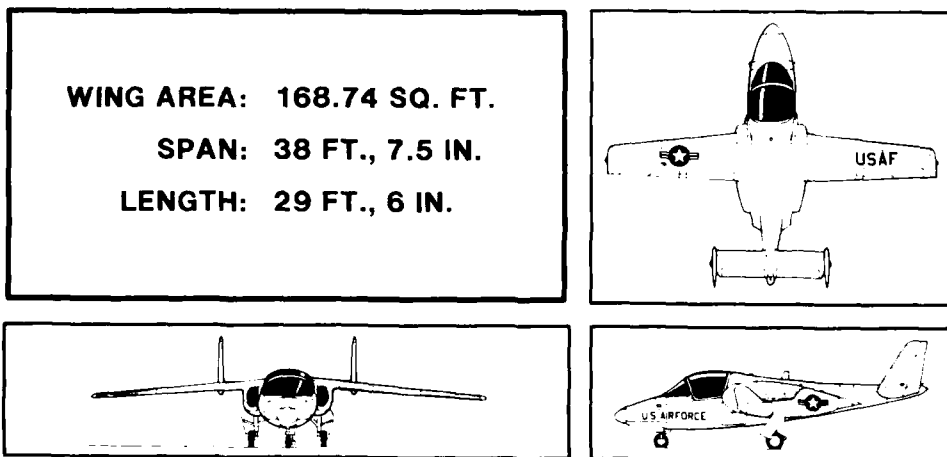
T-46A FIG. 2
