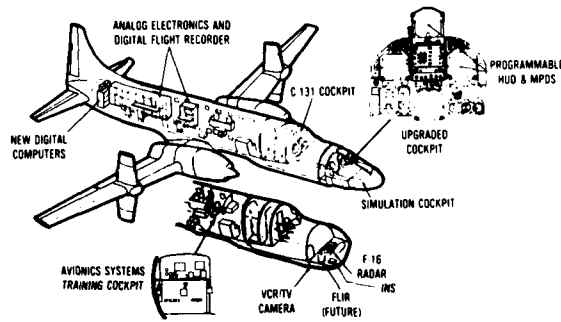
FIG. 11 TIFS MODERNIZATION
