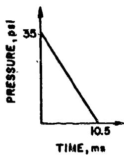
BLAST LOAD
