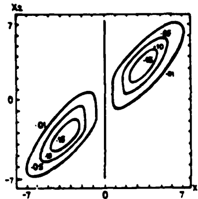
(d) \rho = .9
