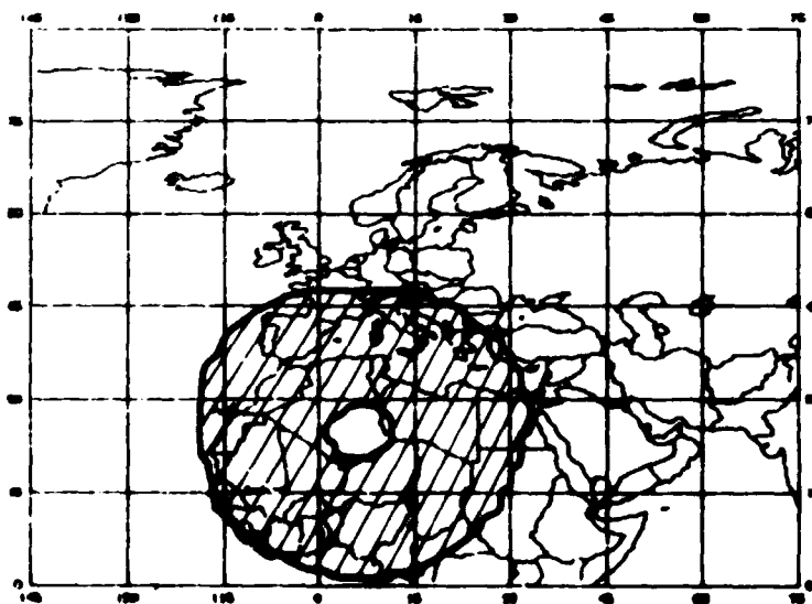
FIG. 2 - COVERAGE AT SATELLITE LONGITUDE 7°
