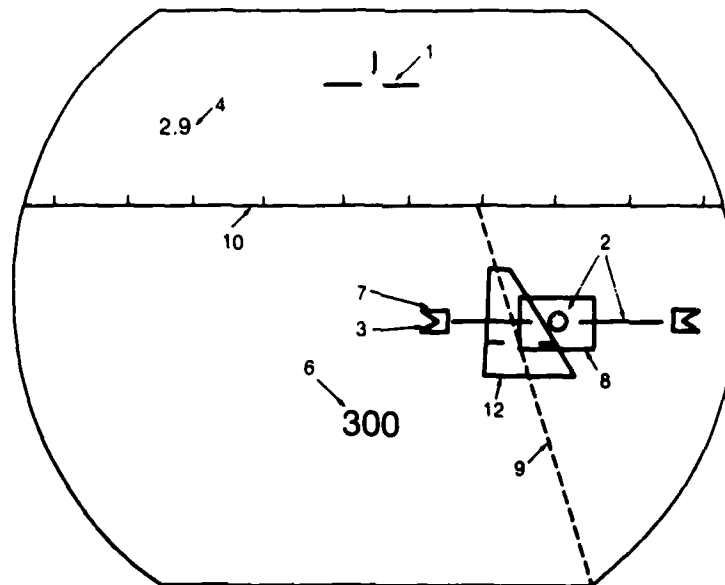
Fig. 10 PERSEPOLIS MLS symbology on HUD /7/
