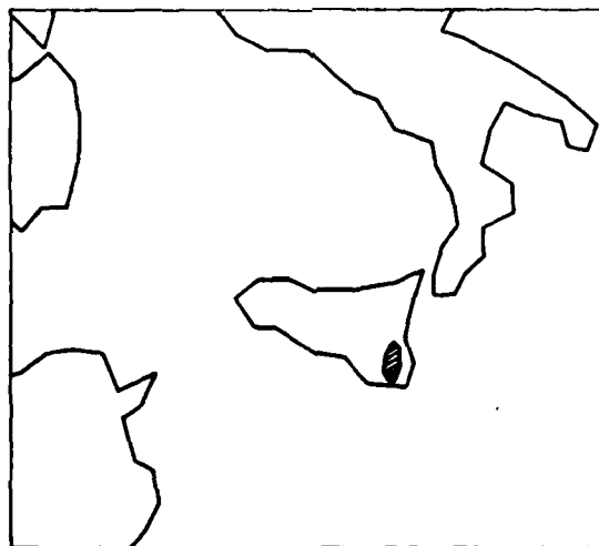
FIG. 6 - TYPICAL FOOTPRINT AT SATELLITE LONGITUDE 17°
