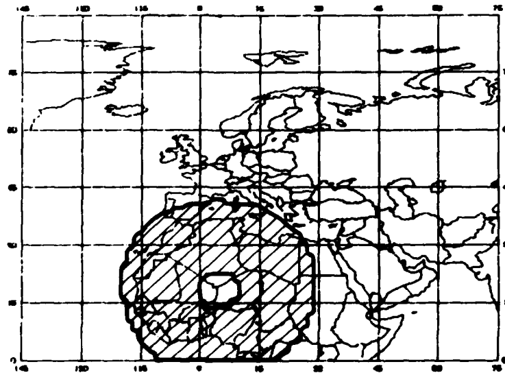
FIG. 1 - COVERAGE AT SATELLITE LONGITUDE 5°
