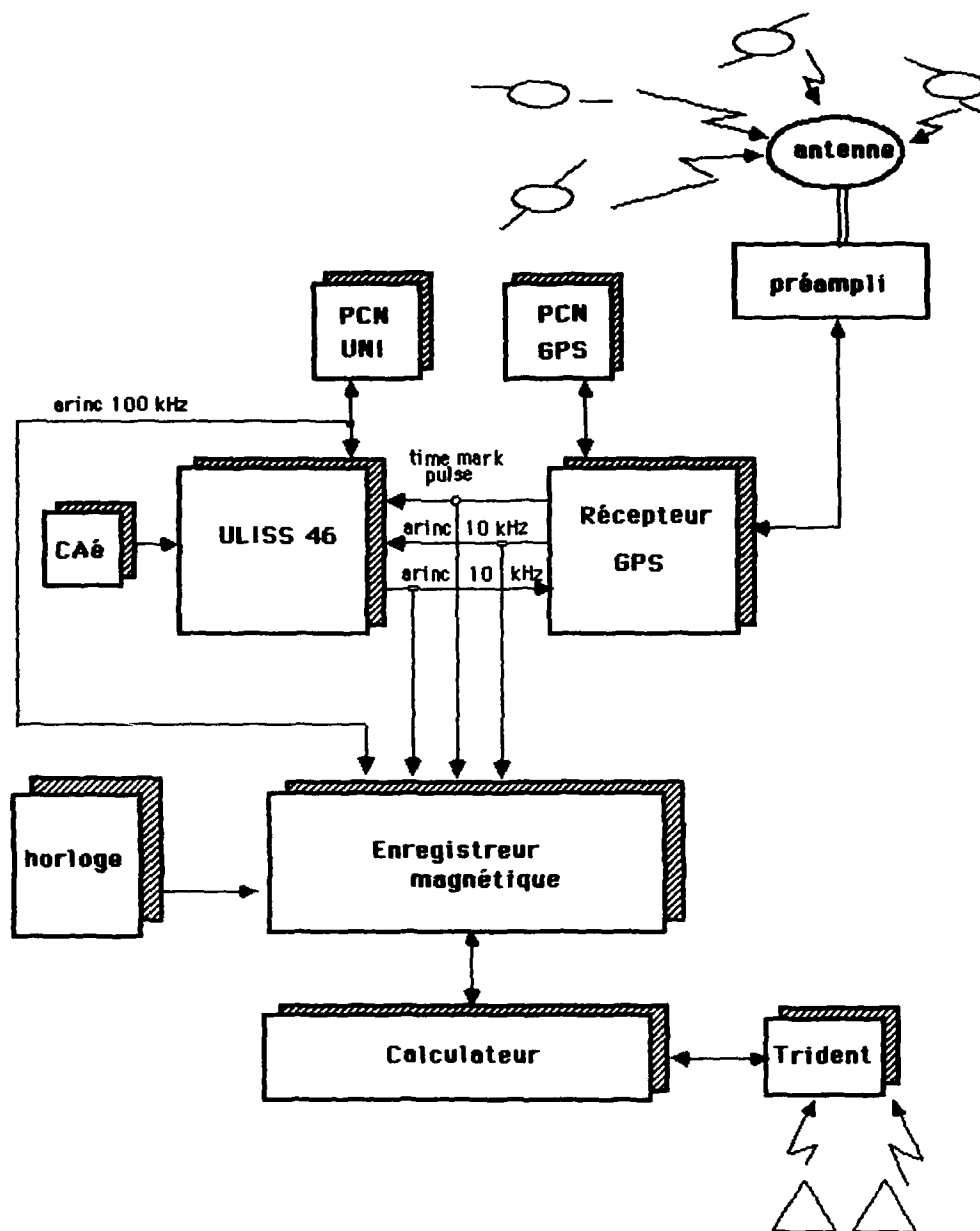
Configuration avion du couplage inertie/gps
