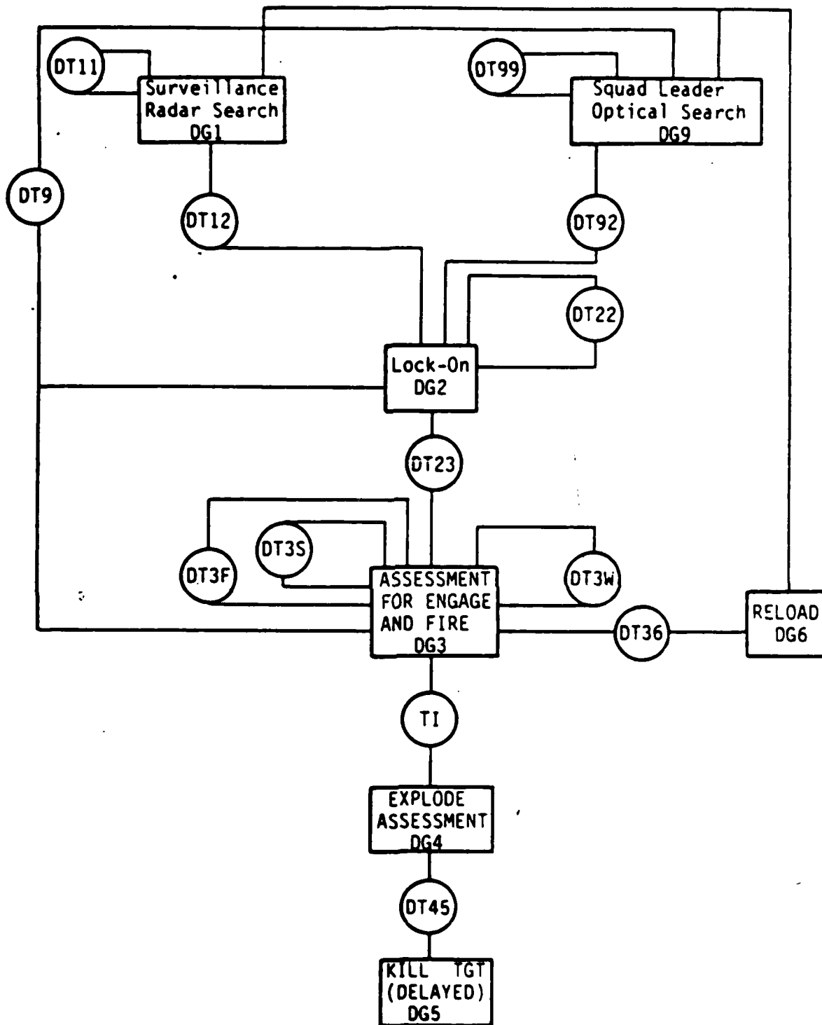
Figure 3. SGT YORK COMO III MODEL
