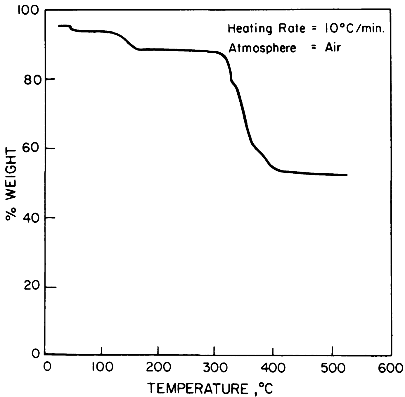
Figure 1. Thermogram of 100\text{Li}_2\text{B}_4\text{O}_{13} \cdot 4\text{Li}_2\text{CO}_3 \cdot 8\text{H}_2\text{O} .
