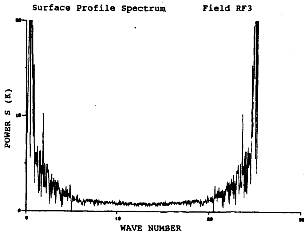
Figure 20 (d). Site RF3 - Grass Field
