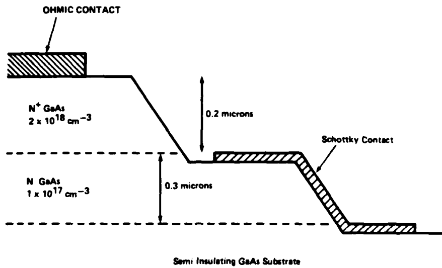
FIG 1 FET TYPE MATERIAL STRUCTURE
