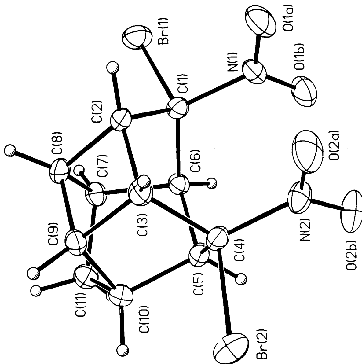
8,11-Dibromo-8,11-dinitro-pentacyclo[5.4.0.0 2,6 .0 3,10 .0 5,9 ]undecane
