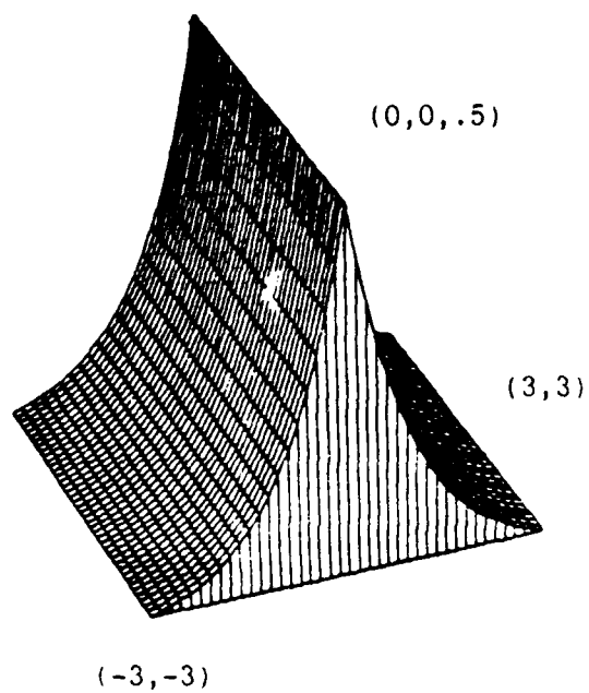
Fig. 9a. Conditional Exponential pdf, \rho=0
