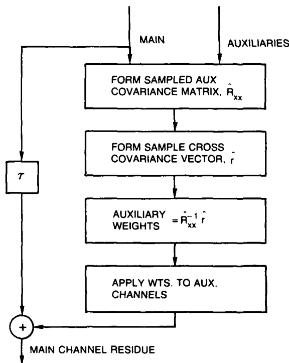
Fig. 3 — SMI canceller
