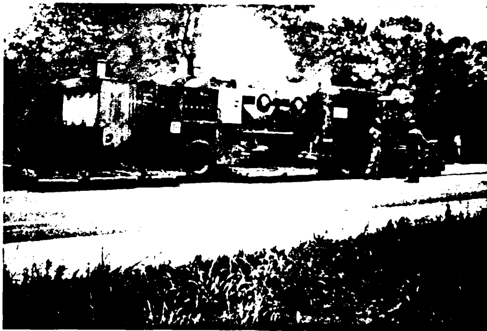
b. Wirtgen Repaver/Remixer
