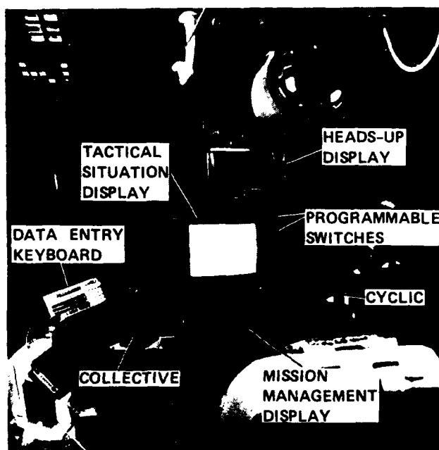
Fig. 3 SPACES cab.
