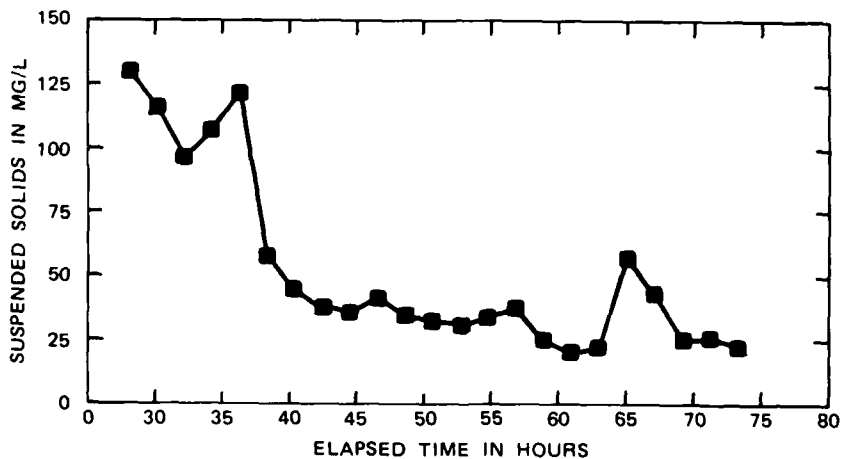
b. Effluent
