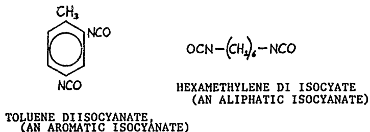
Fig. 57a. TYPICAL DI ISOCYANATES
