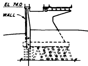
SECTION D-D
