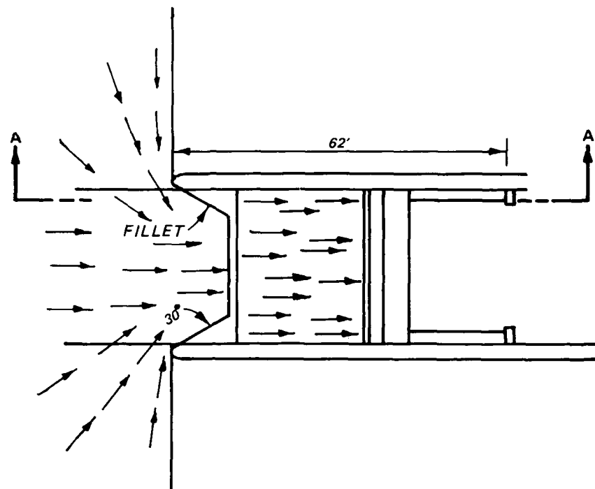
a. Plan
