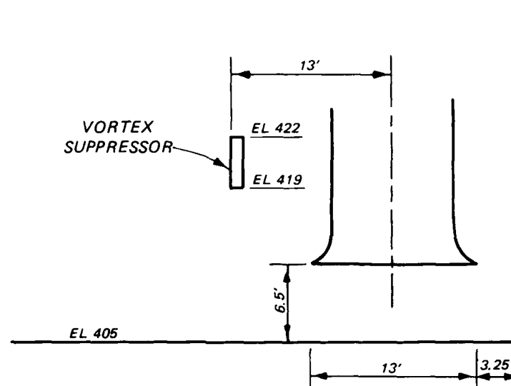
a. Elevation
