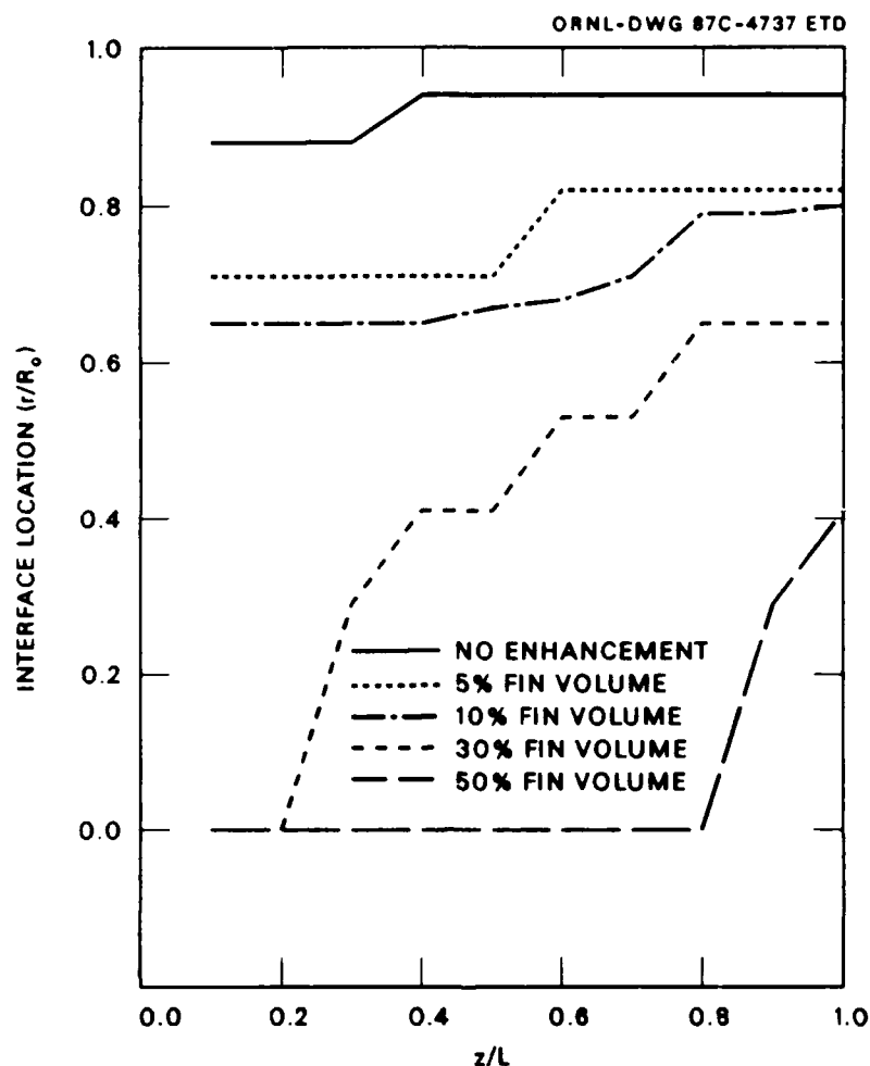
Fig. 4.8. Phase-Change Front Positions for 304SS Thin Fin Enhancements.
