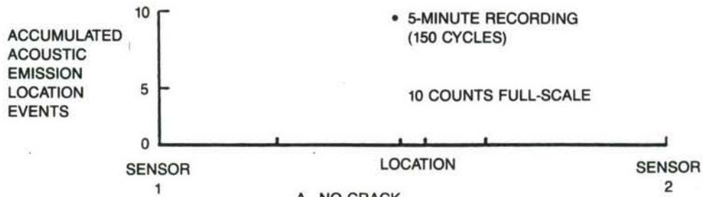
A. NO CRACK
