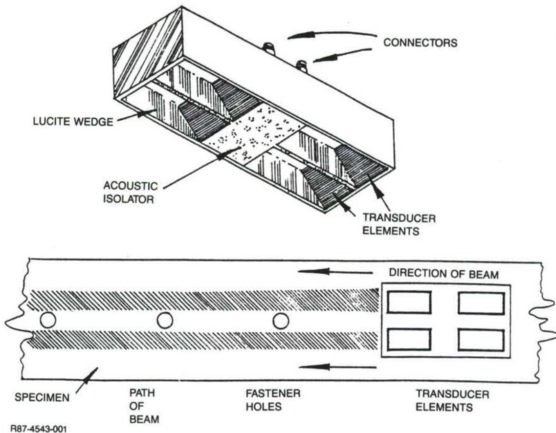
Fig. 1 Ultrasonic Array
