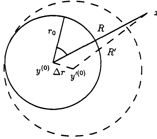
Figure 3.2: Lemma 3.2.1
