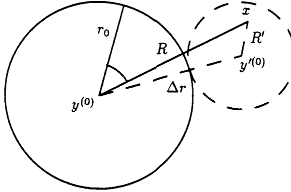
Figure 3.3: Lemma 3.2.2
