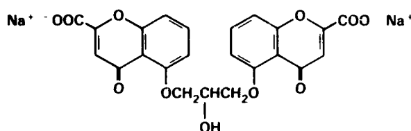
Fig. 1. Disodium cromoglycate (DSCG).
