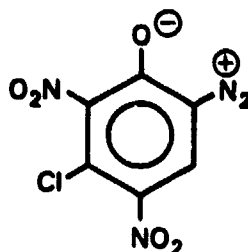
5-Cl-DDNP
