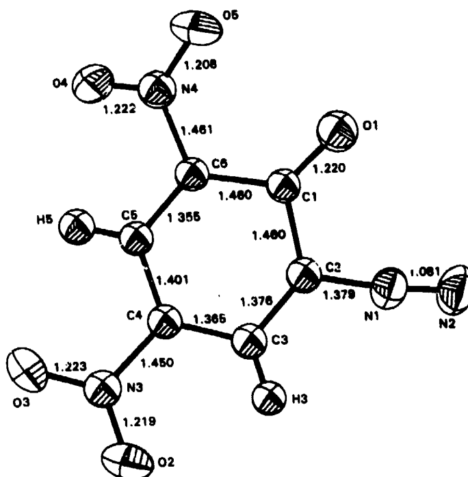
DDNP
