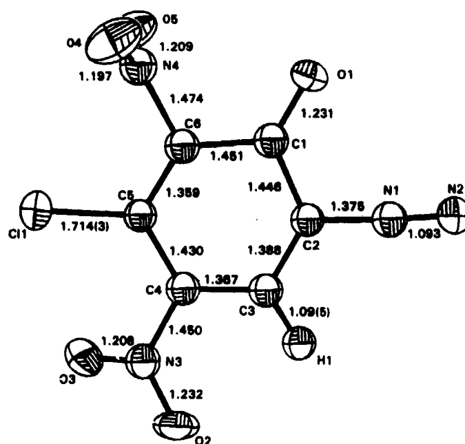
5-Cl-DDNP
