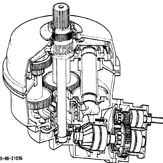
(d) 500-hp BEARINGLESS PLANETARY (HIGH-RATIO).
