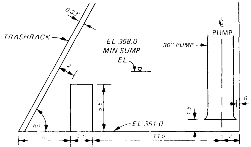
b. ELEVATION
