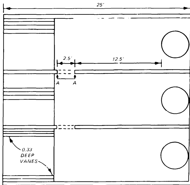
a. PLAN
