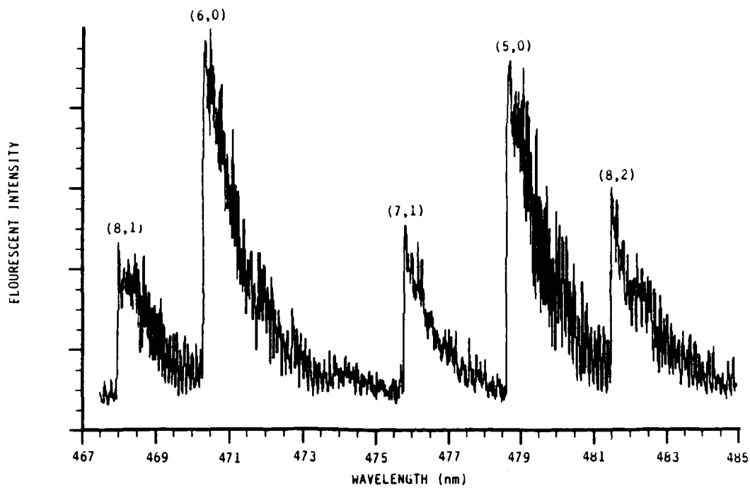
(b) Coumarin 480
