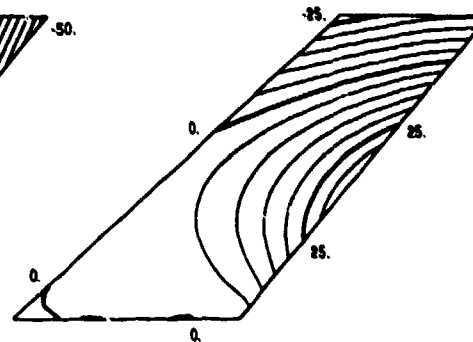
(d) Node 3, f_3 = 48.3482 Hz
